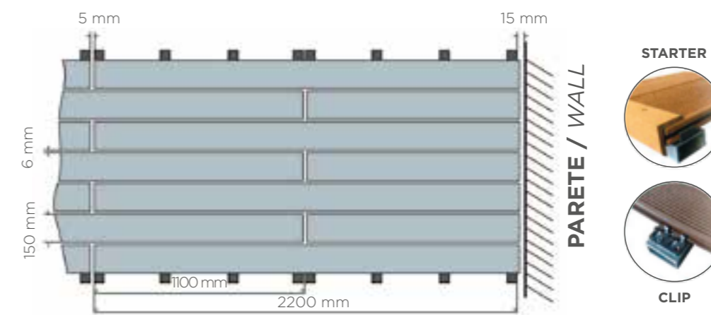
SCHEMA DI POSA WPC / INSTALLATION DIAGRAM
